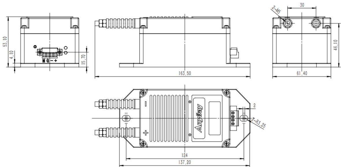
图 1 外形尺寸图
