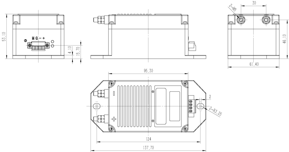
图 1 外形尺寸图
