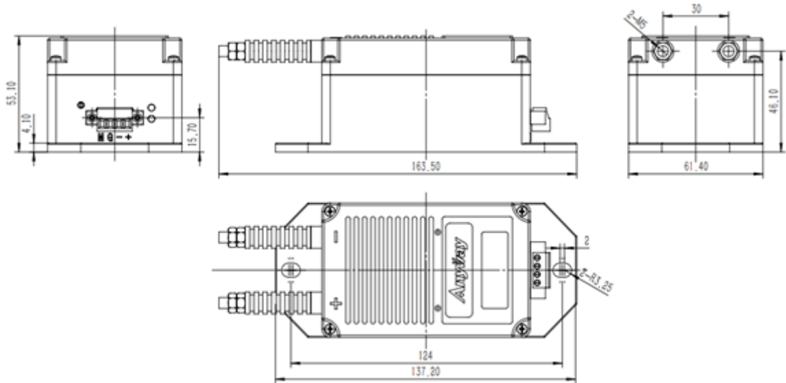
图 1 外形尺寸图
